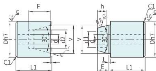
组装尺寸
