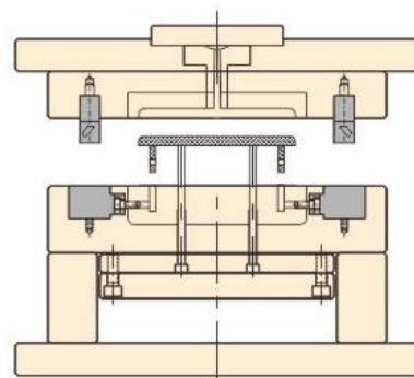
开模状态
