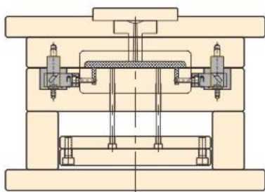
合模状态
