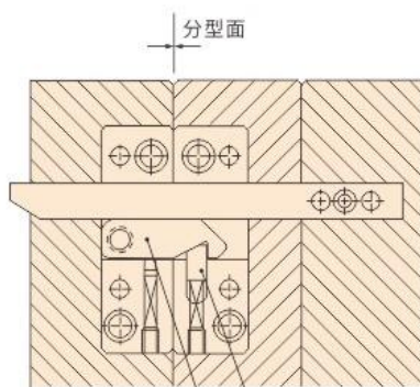
凸轮锁块 锁紧块 合模状态
