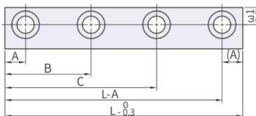
螺栓孔规格表
