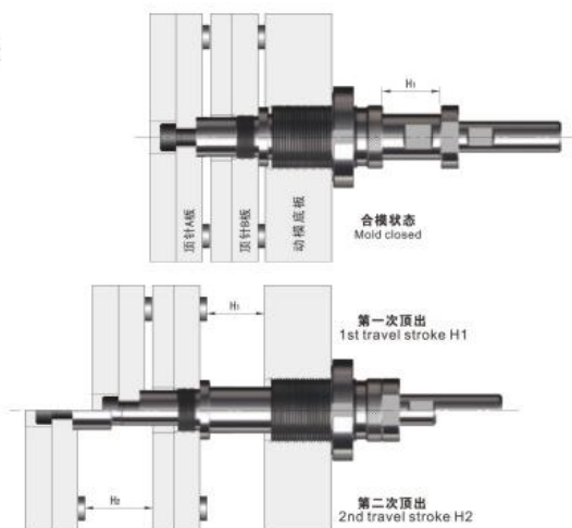
功能示意图 Functional chart
