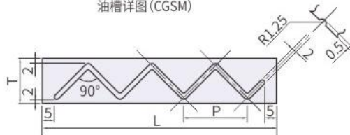
油槽详图 (CGSM)
