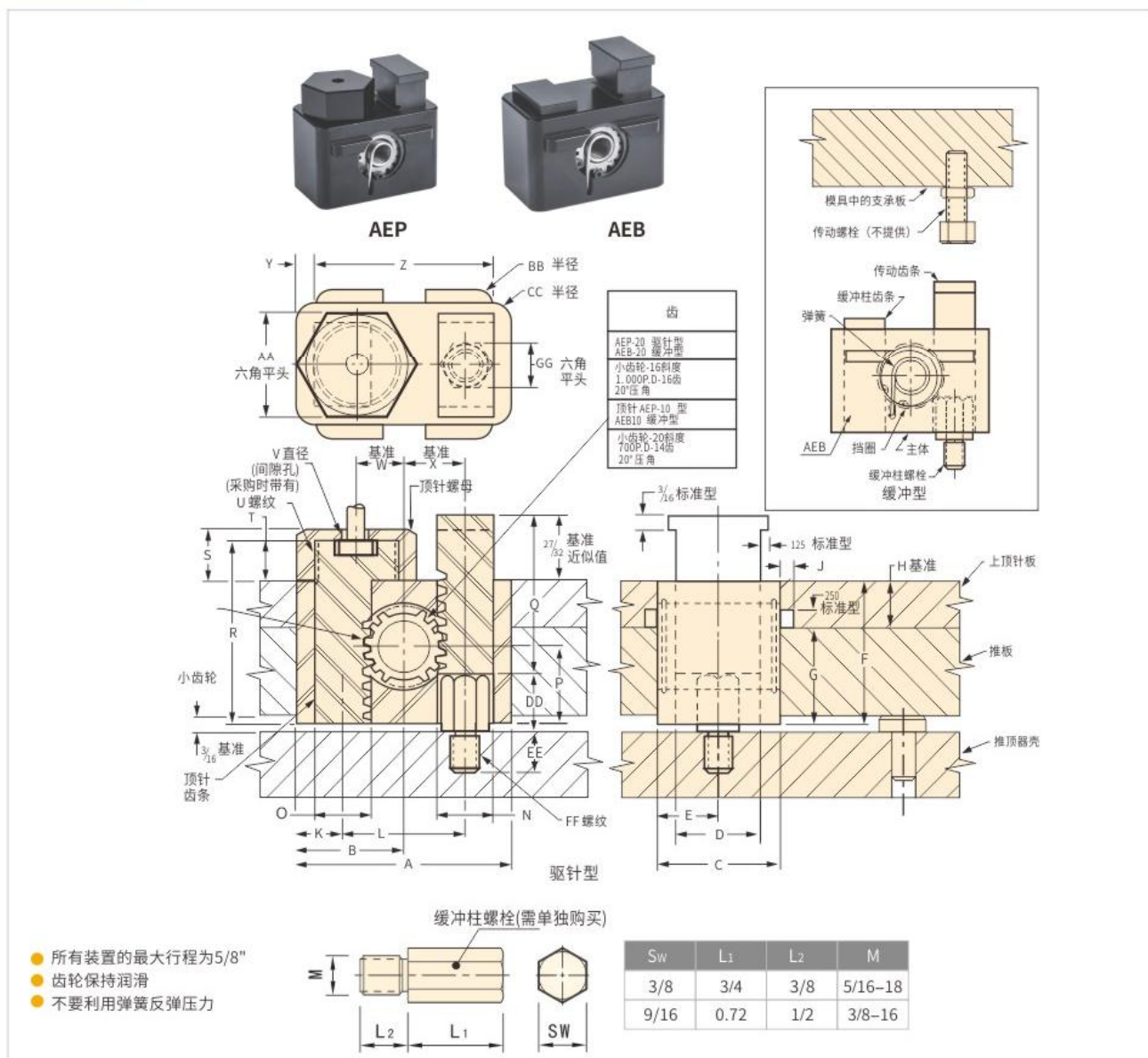
加速顶出器尺寸
