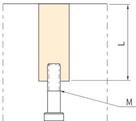
日期章与模具上的孔需顺配安装
