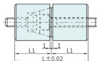
组装尺寸
