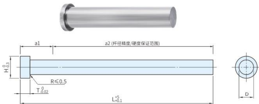
杆径D公差
