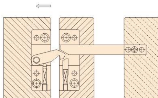
开模中
