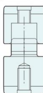
合模开始导向定位
