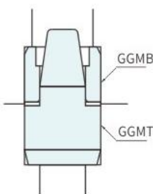
导柱·导套安装范例
