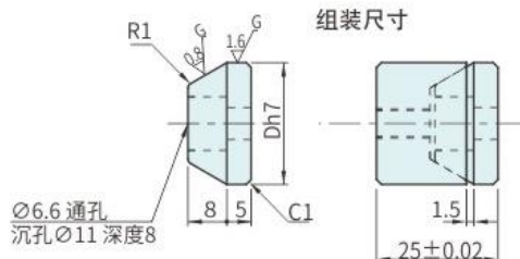
组装尺寸
