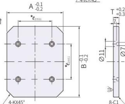
4螺栓孔型 A>40, B≥80时
