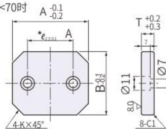
2螺栓孔型 A>40, B<70时
