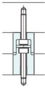
安装效果图
