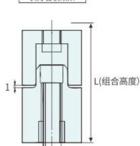
实际合模效果
