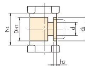
截面 A-A
