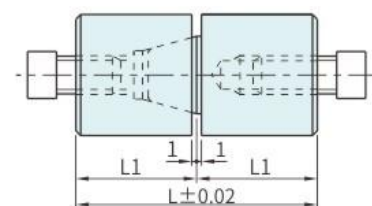
组装尺寸
