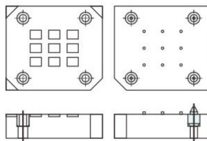
导柱·导套使用范例
