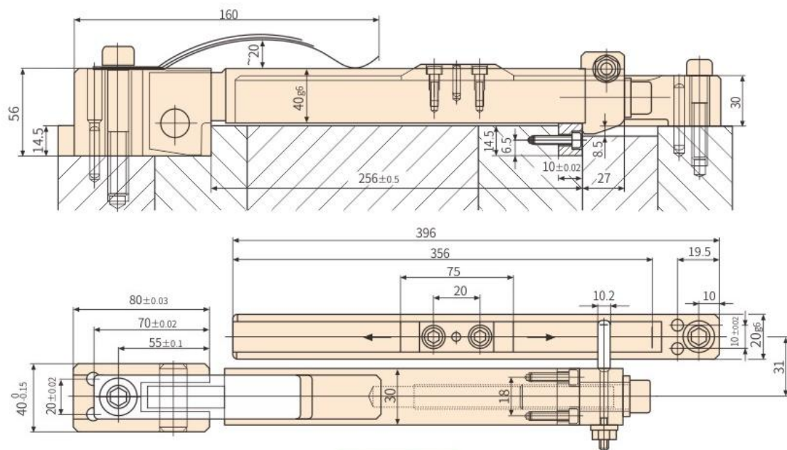
ZZ5-2尺寸图
